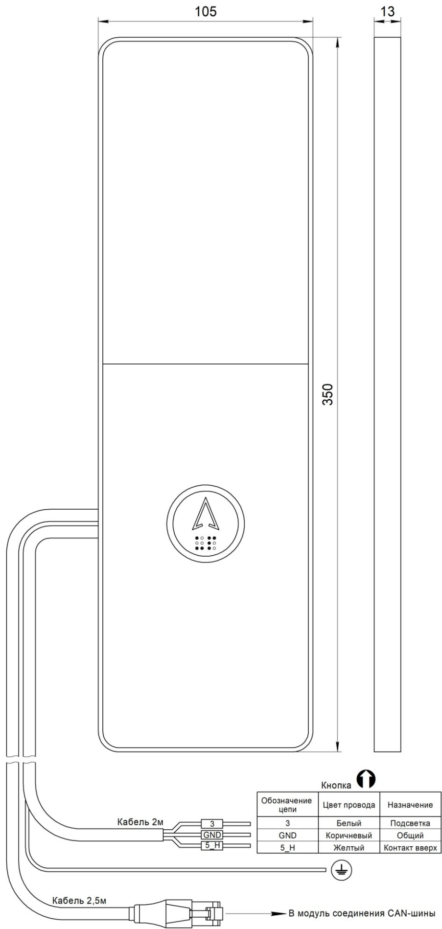
Рис.1 Внешний вид, габаритные и установочные размеры Вызывного поста МАЛАХИТ (жгут RJ45) НШЕК.468381.015
